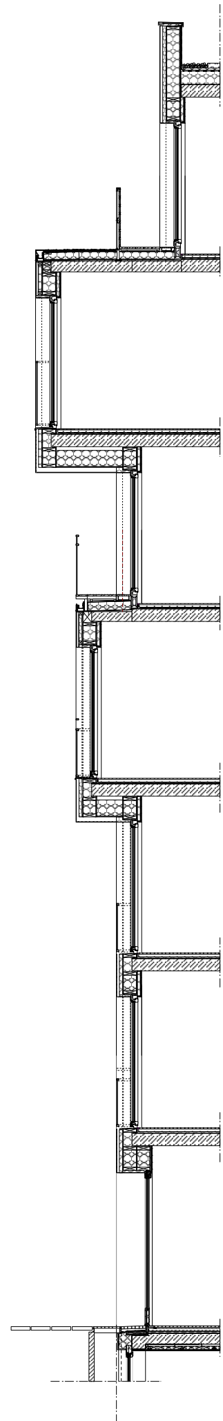
Der Schnitt durch die Nordfassade verdeutlicht die wärmebrückenfreie Ausführung der Außenhülle.
